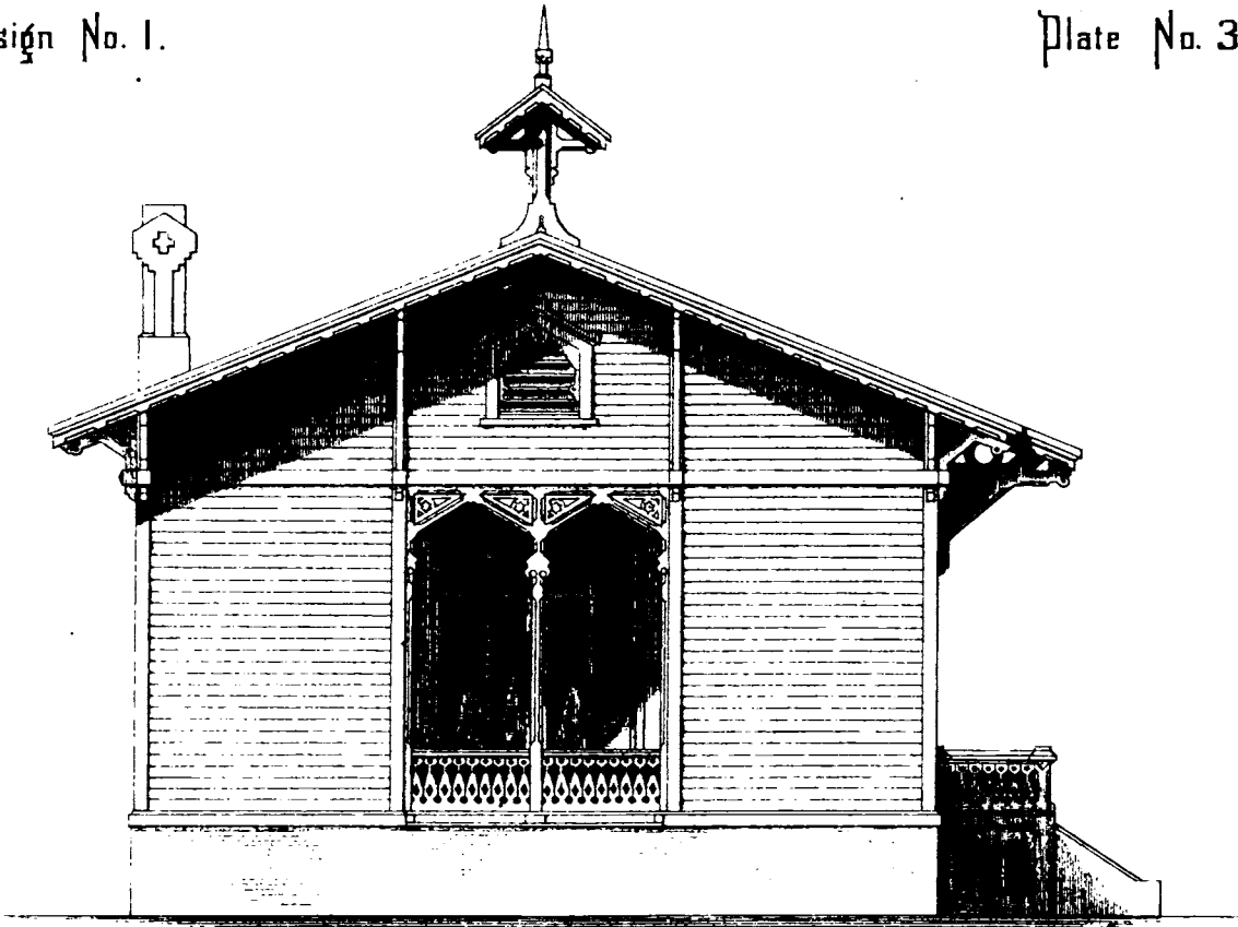
END ELEVATION
