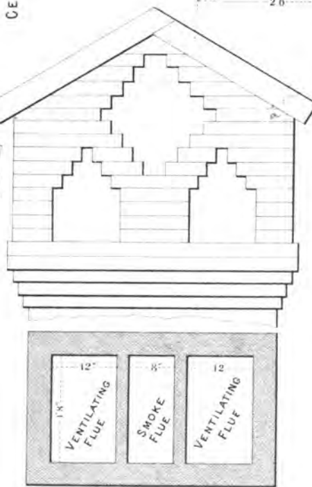
CHIMNEY TOP
