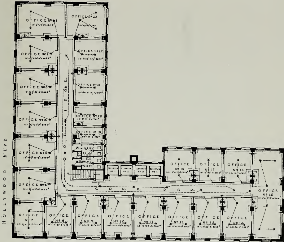
VINE STREET · · · · · TYPICAL FLOOR PLAN · · · · · TOTAL RENTABLE FLOOR AREA = 7200' · SCALE 1/8" = 1'-0"
