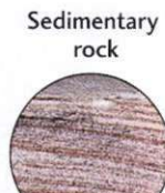
Sediment
