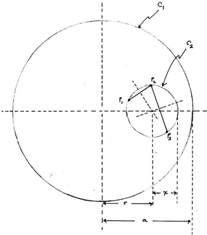
Fig. 1.8.1 A ‘Circle Inside A Circle’
