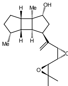
(+)-Spatol
