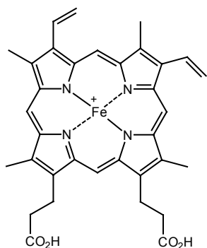
Hemin (Fischer, 1929)
