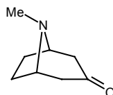
Tropinone (Robinson, 1917)
