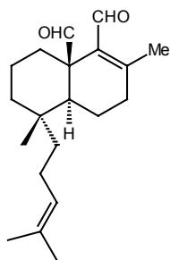
(+)-Perrottetinal A
