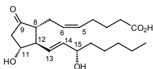
PGE 2
