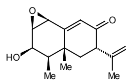
Eremofortin B
