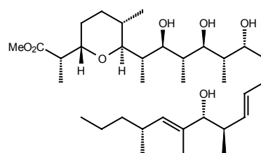
(+)-Zincophorin
