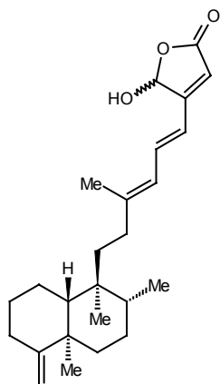
Palauolide
