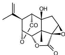
Picrotoxinin
