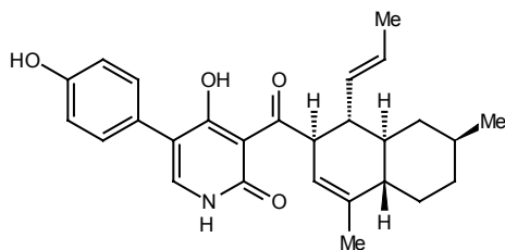
Illicolin H
