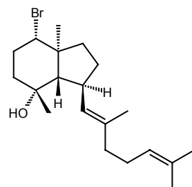
Prepinnaterpene
