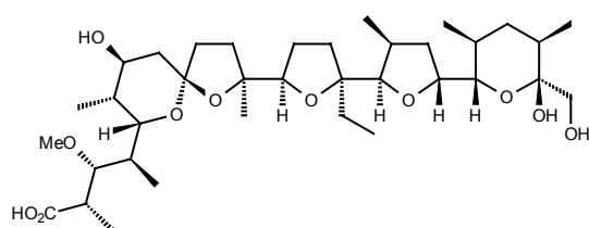
Monensin
