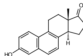
Equilenin (Bachmann, 1939)
