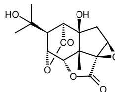
Picrotin
