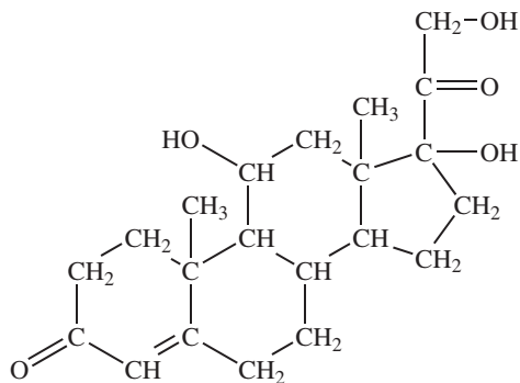
Cortisol
