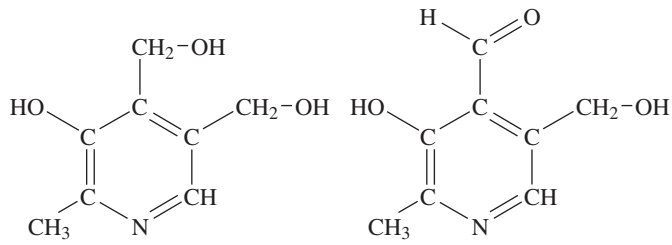
Pyridoxine
