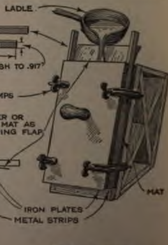
Fig. 5: POURING
