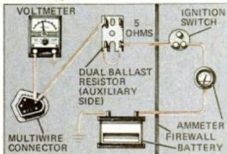
Test No. 3: Voltage should be \pm 1 volt.
