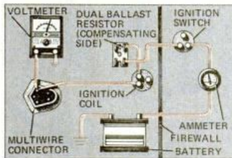
Test No. 2: Voltage should be \pm 1 volt.
