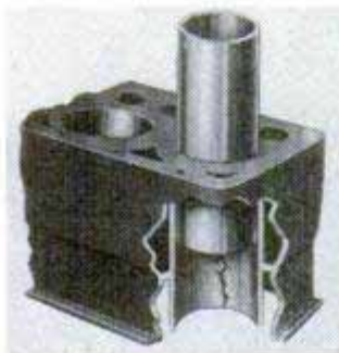
Fig. 1—Dry sleeve
