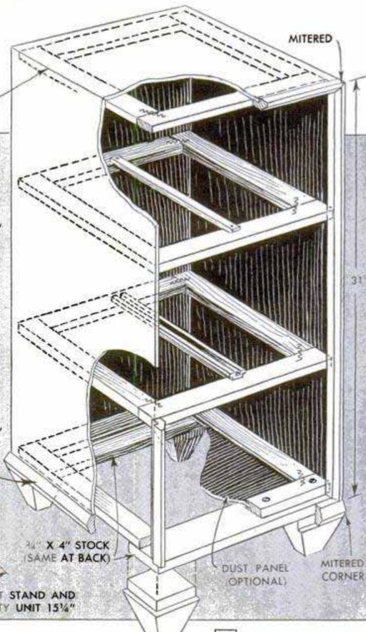
NIGHT STAND
