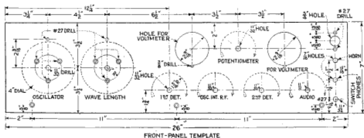
FRONT-PANEL TEMPLATE
