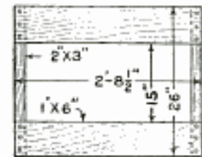
DADO TABLE AND GUIDE Fig. 6
