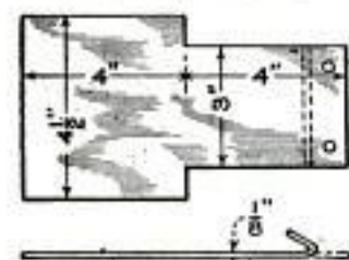
FAN BLADE, 6 REQUIRED
