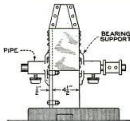
END ELEVATION
