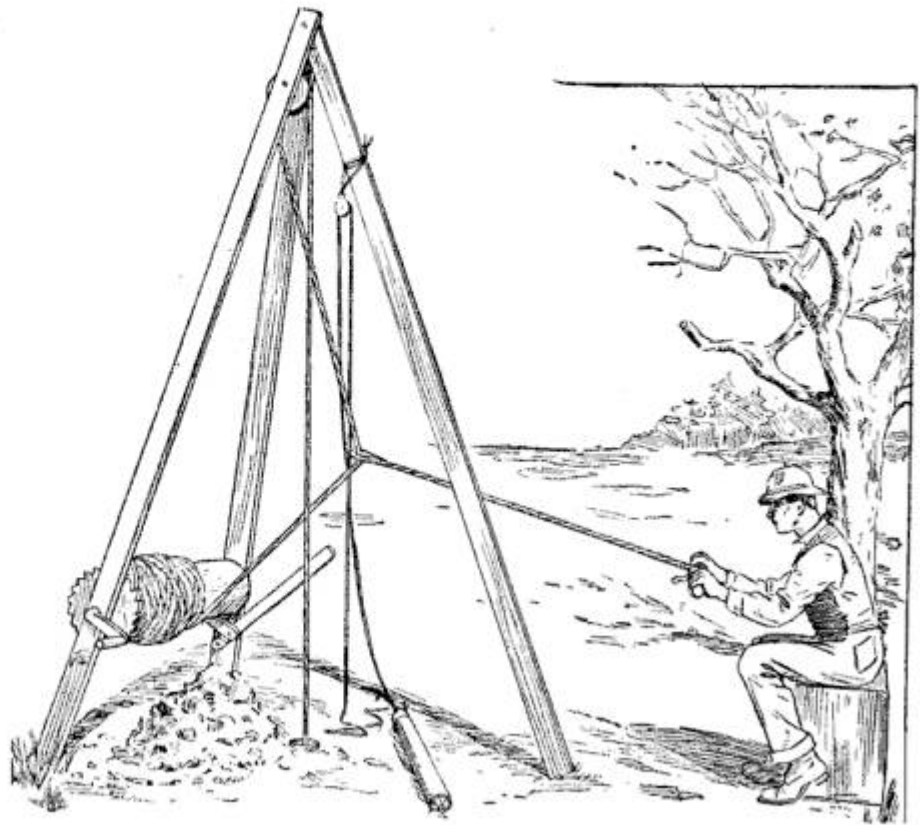
Fig. 2—The Derrick
