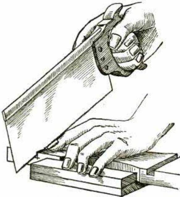
Fig. 70—Sawing Dado
