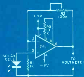
Fig. 1. Light meter circuit.
