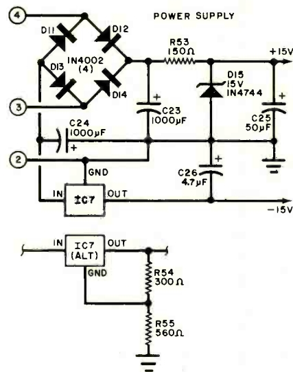
Fig. F. Power-supply circuit.
