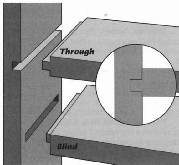
Tongue-and-Dado
