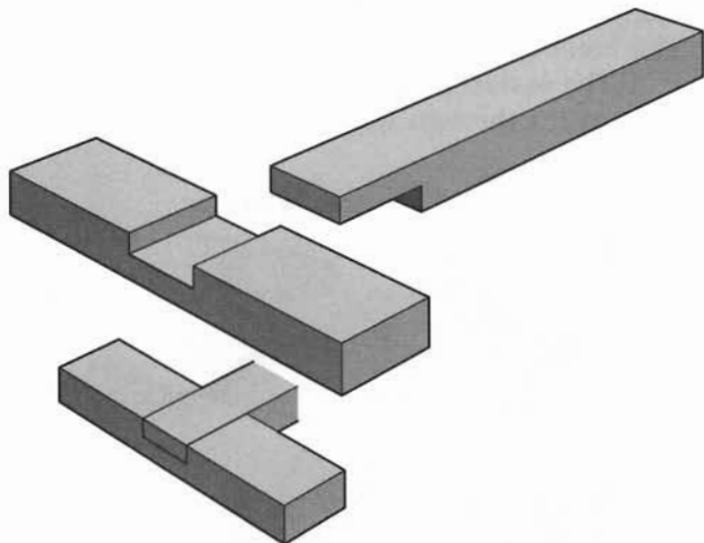
T-Lap
