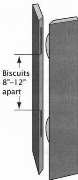
Biscuited Edge Miter
