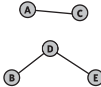
(e) Add edge (D,E), weight=2
