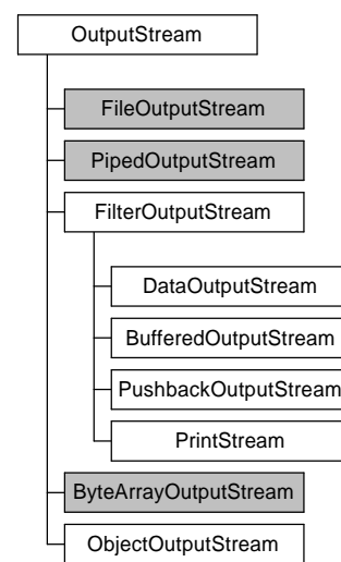
Figura 9.2. Jerarquía de clases OutputStream.
