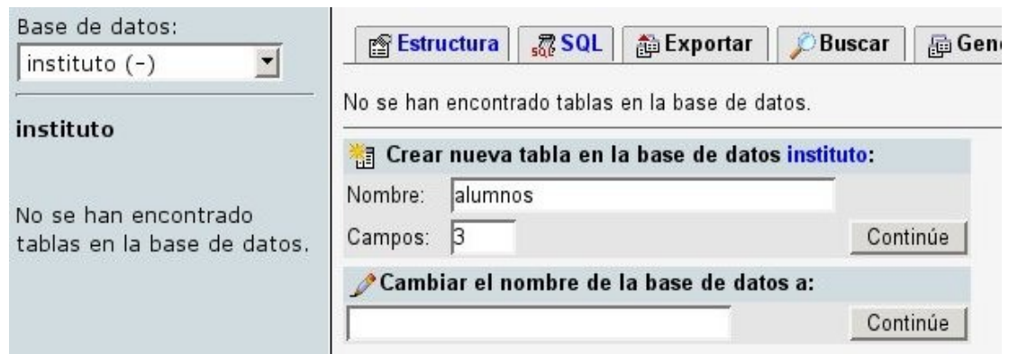
8.16.5. listado.php
