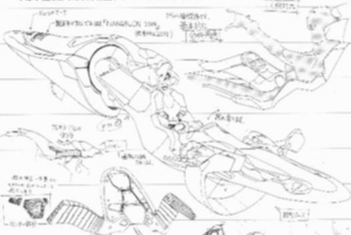
◆◆右前方から。上は、ほぼ決定稿に近い状態のラフ。やはり後方部の形状が煮詰まっていなのがわかる
