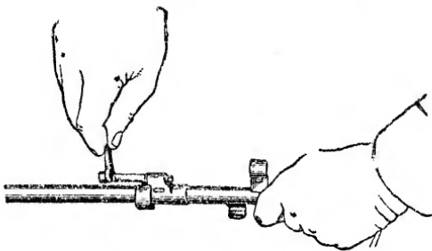
Рис. 70. Отделение патрубкa
