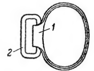
Рис. 51. Ложевое кольцо: 1 — прилив; 2 — кольцо для винтовочного ремня
