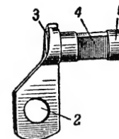
Рис. 38. Предохранитель: 1 — стержень; 2 — флажок; 3 — выступ головки; 4 — вырез для головки упора
