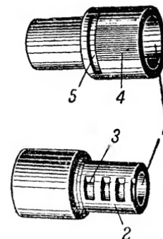
Рис. 16. Втулка ствольной коробки:
