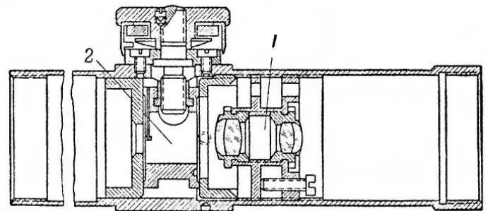
Рис. 98. Разрез корпуса прицела: 1 — оборачивающая система; 2 — механизм установки углов прицеливания и боковых поправок
