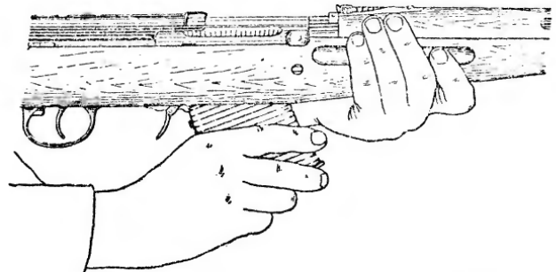
Рис. 56. Отделение магазина от ствольной коробки
