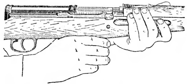
Рис. 55. Отделение магазина от ствольной коробки
