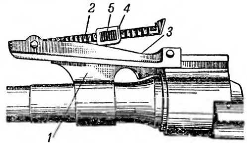
Рис. 10. Прицел:
