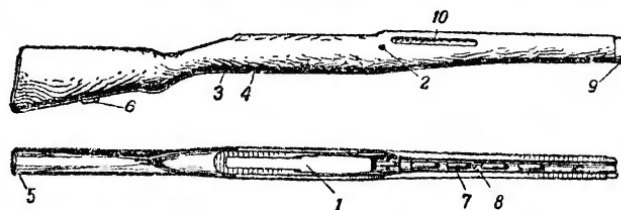
Рис. 46. Ложа:
