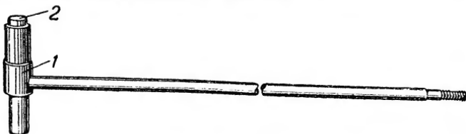
Рис. 89. Шомпол: 1 — рукоятка; 2 — шомпольный упор
