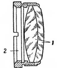
Рис. 97. Разрез объектива: 1 — линзы; 2 — оправа
