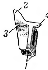
Рис. 19. Отражатель: 1 — боковые выступы; 2 — верхний выступ; 3 — ограничительный выступ; 4 — задний выступ; 5 — паз.
