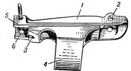
Рис. 11. Колодка прицела:
