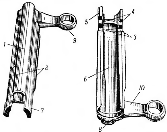
Рис. 26. Стебель затвора: 1 — гребень; 2 — направляющие выступы; 3 — нижние вырезы; 4 — срезы; 5 — выступ; 6 — жолоб; 7 — задний вырез; 8 — гнездо; 9 — рукоятка; 10 — номер.
