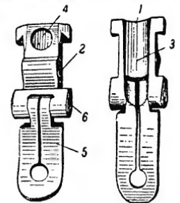
Рис. 39. Защелка магазина: 1 — верхний срез; 2 — отверстие для оси; 3 — полукруглый вырез; 4 — гнездо; 5 — хвост; 6 — ось хвоста
