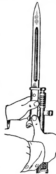
Рис. 73. Примыкание штыка
