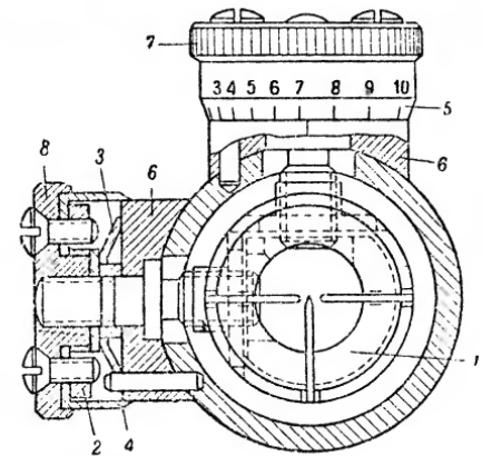
Рис. 100. Механизм установки углов прицеливания и боковых поправок:
