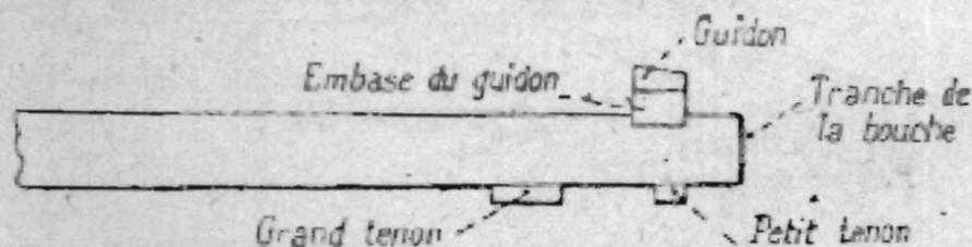
Fig. 2. — Canon (Partie antérieure.)
