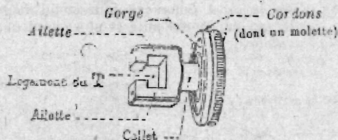
Fig. 12. — Manchon.
