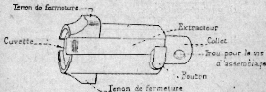
Fig. 7. — Tête mobile.
