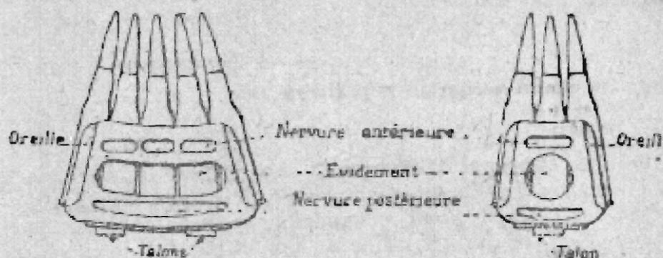
Fig. 15. — Chargeur M n 1916, à 5 cartouches.
