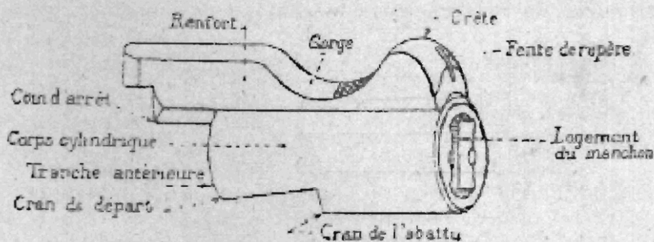
Fig. 10. — Chien.
