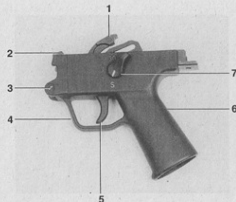
Bild 3 Griffstück mit Abzugsvorrichtung
