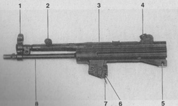
Bild 2 Lauf und Verschlussgehäuse
