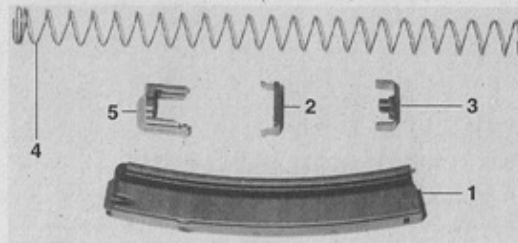
Bild 7 Magazin
