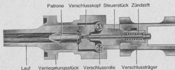
Bild 9 Verschluss geschlossen
