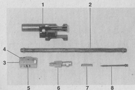
Bild 4 Verschluss
