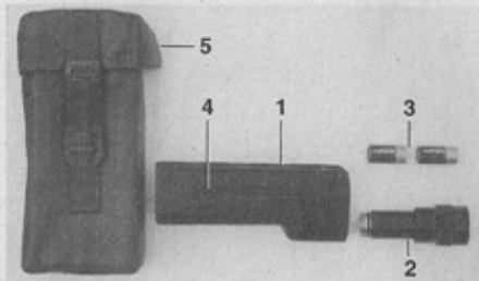
Bild 2 Hauptbestandteile des WLicht Gt
