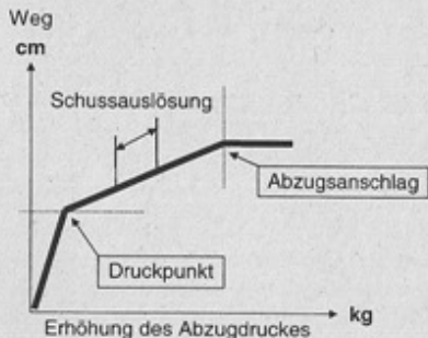
Bild 60 Der Druckverlauf am Abzug im Verhältnis des Weges
