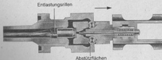
Bild 10 Verschluss geöffnet
