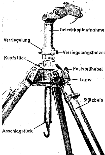
Kopfstück mit Stützbeinen
