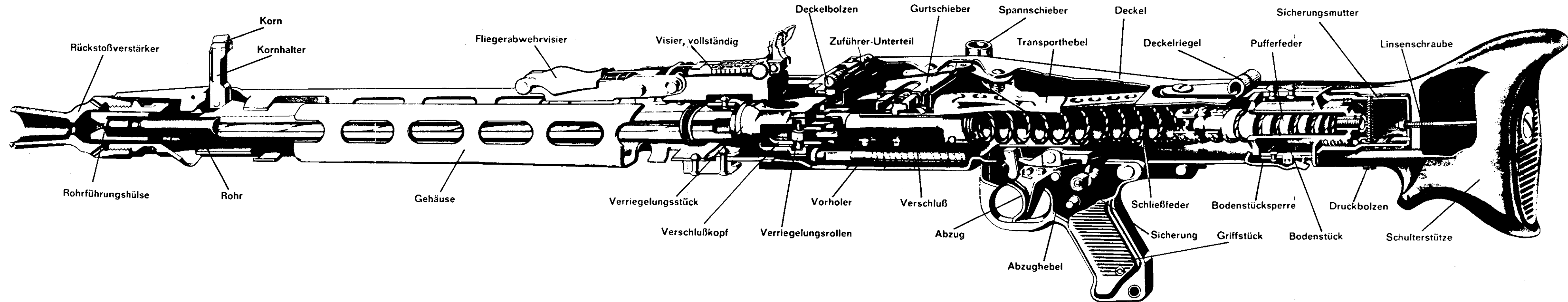
Schnittbild
