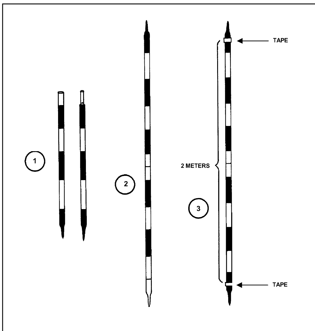
Figure C-7. Subtense bar.
