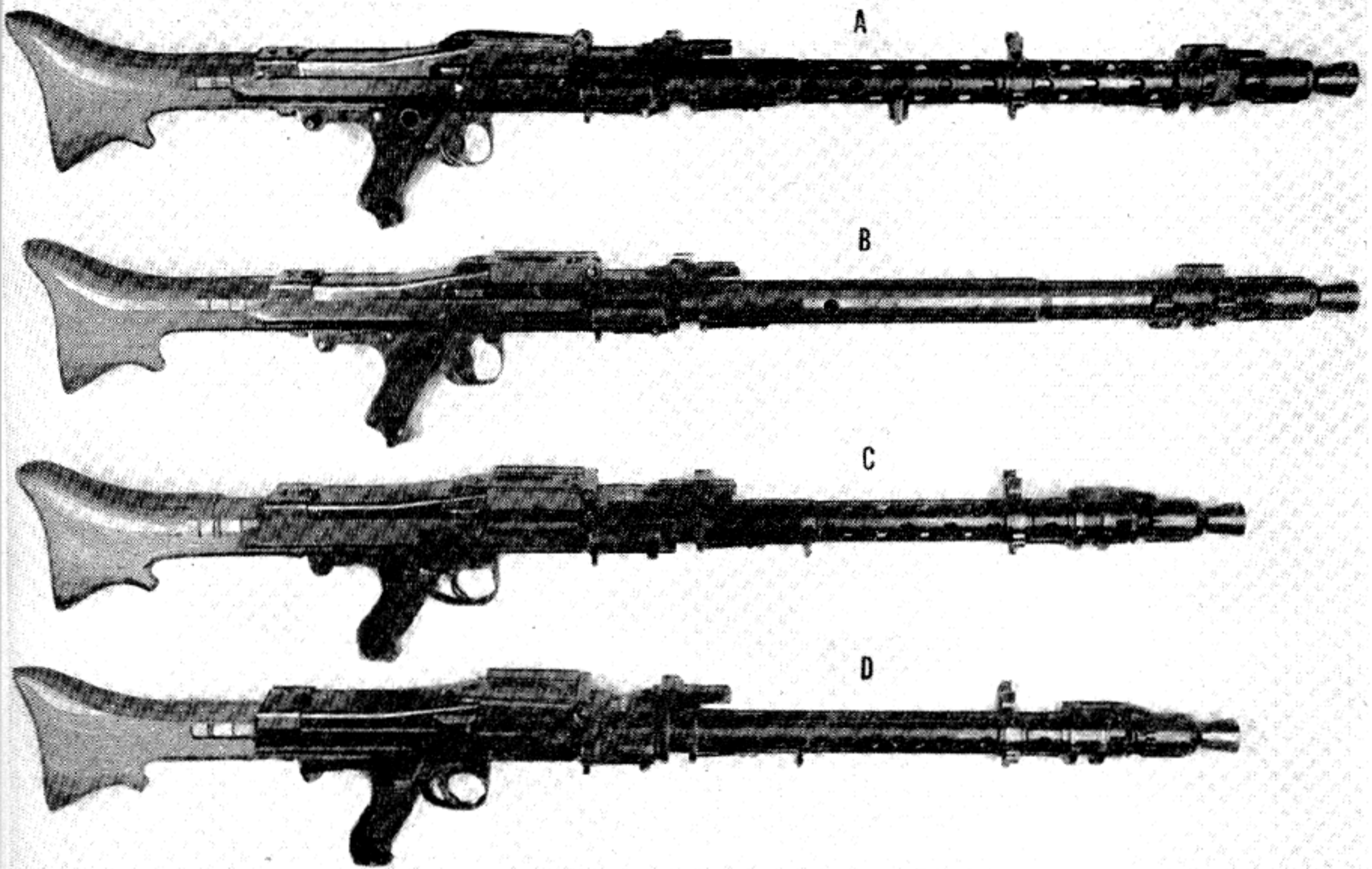
Comparison of Mauser Machine Guns of the MG-34 Series. (A) MG-34. (B) MG-34 (Modified). (C) MG-34 S. (D) MG-34/41
