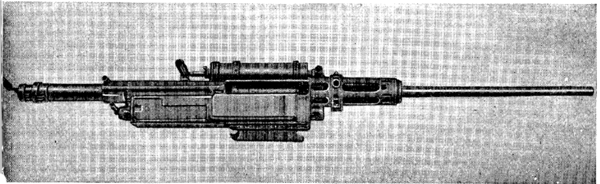
Szakats 20-mm Automatic Aircraft Cannon, Model SZB.
