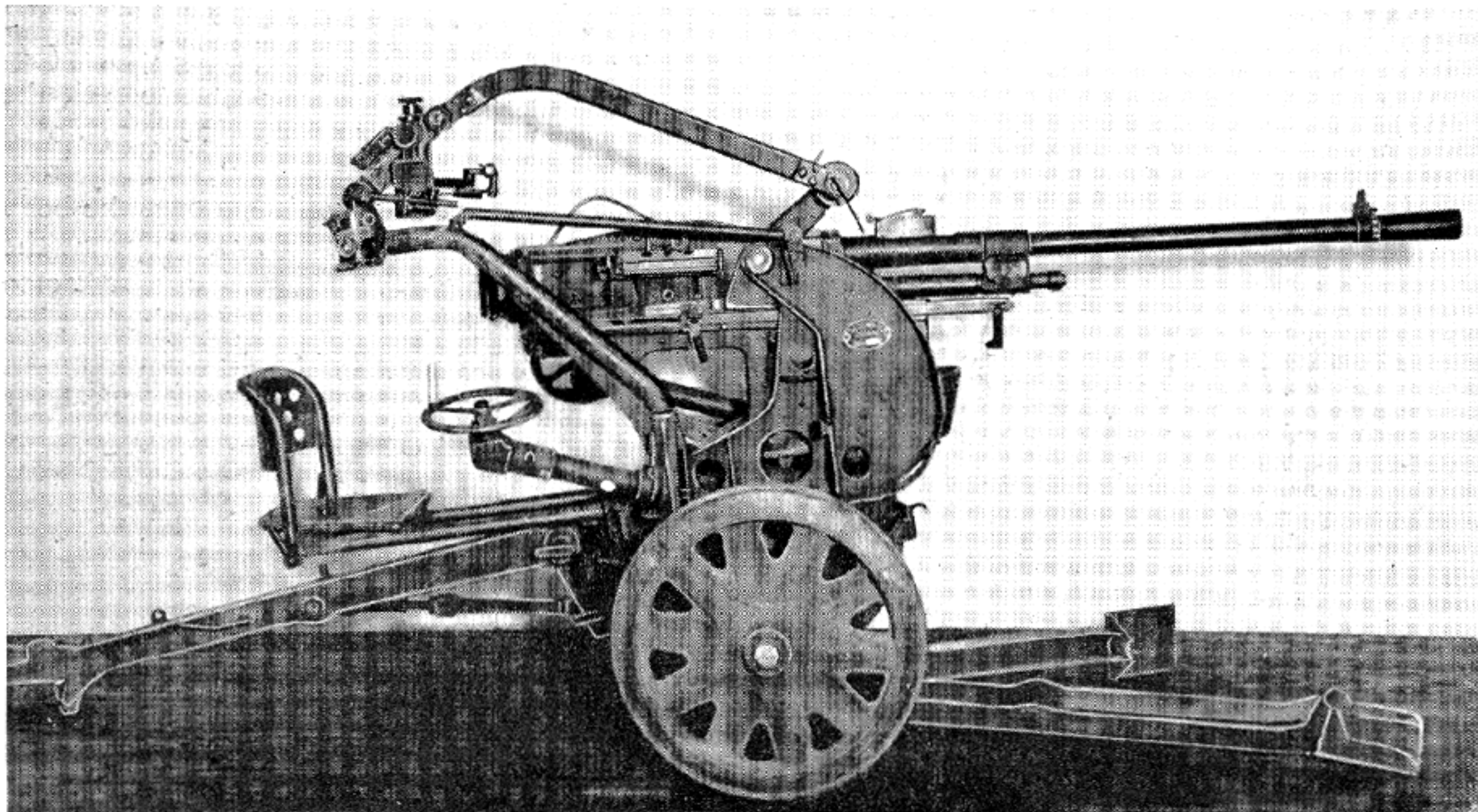
Breda 20-mm Antitank Automatic Cannon.
