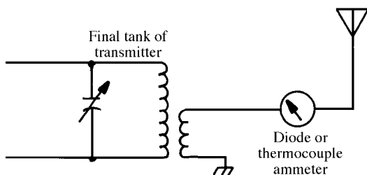
antenna ammeter
