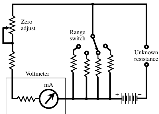
ohmmeter
