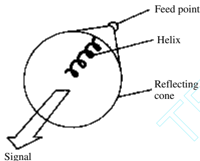
helicone
