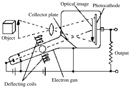
iconoscope
