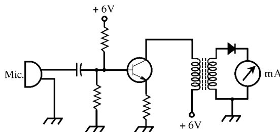
applause meter
