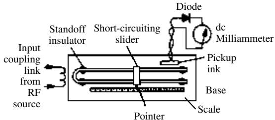
Lecher frame
