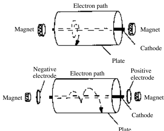
end-plate magnetron
