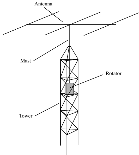
rotatable antenna
