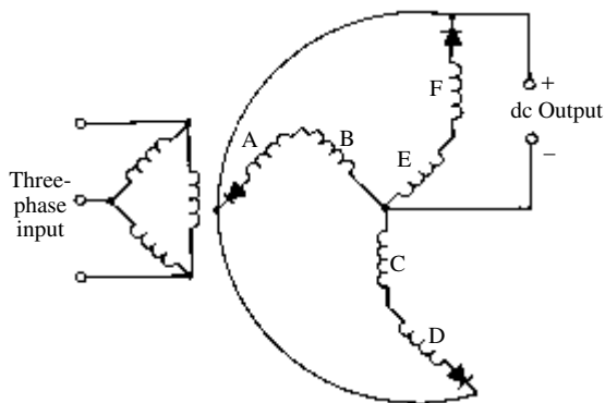
zigzag rectifier
