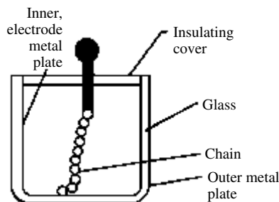
Leyden jar
