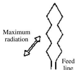
Chireix-Mesny antenna
