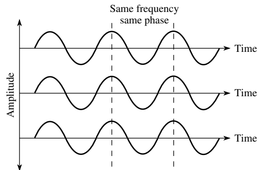
coherence
