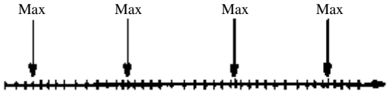
longitudinal wave
