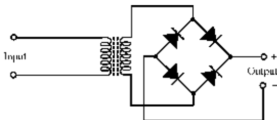
bridge rectifier
