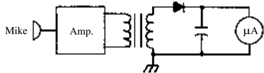
noise meter
