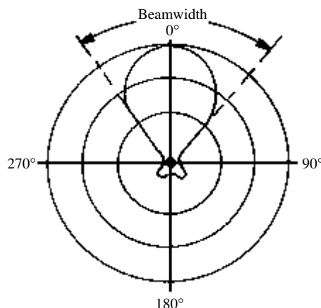
horizontal beamwidth
