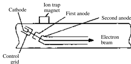
bent gun
