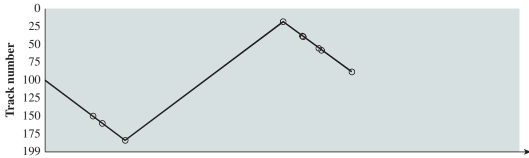
(d) C-SCAN
