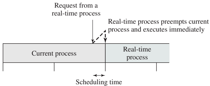
(d) Immediate preemptive scheduler
