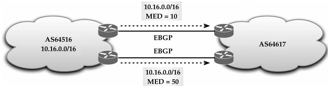
FIGURE 8.8 BGP path attribute: MED example.
