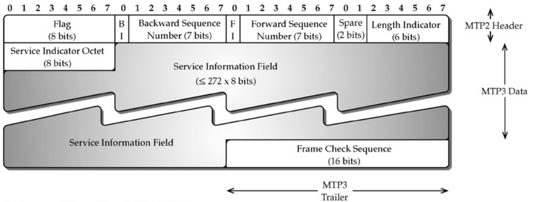
(c) Message Signaling Unit (MSU)
